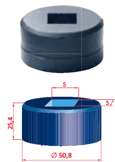
Vierkantmatrize Nr. 03 Art.-Nr. PH-2203
