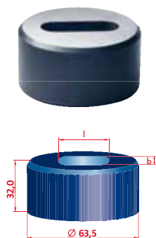
Langlochmatrize Nr. 04 Art.-Nr. PH-2104
