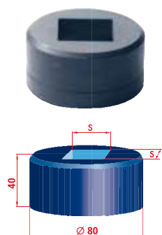
Vierkant-Matrize Nr. 80 Art.-Nr. MU-7204
