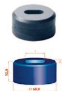
Langlochmatrize Nr. 08 Art.-Nr. GE-2108
