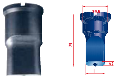
Langlochstempel Nr. 06 Art.-Nr. PH-1106
